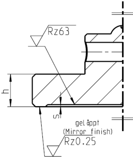
Abbildung 18.1: Stahlteller
